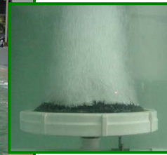
เครื่องเติมอากาศแบบหัวกระจายอากาศใต้น้ำ (Diffuser)
